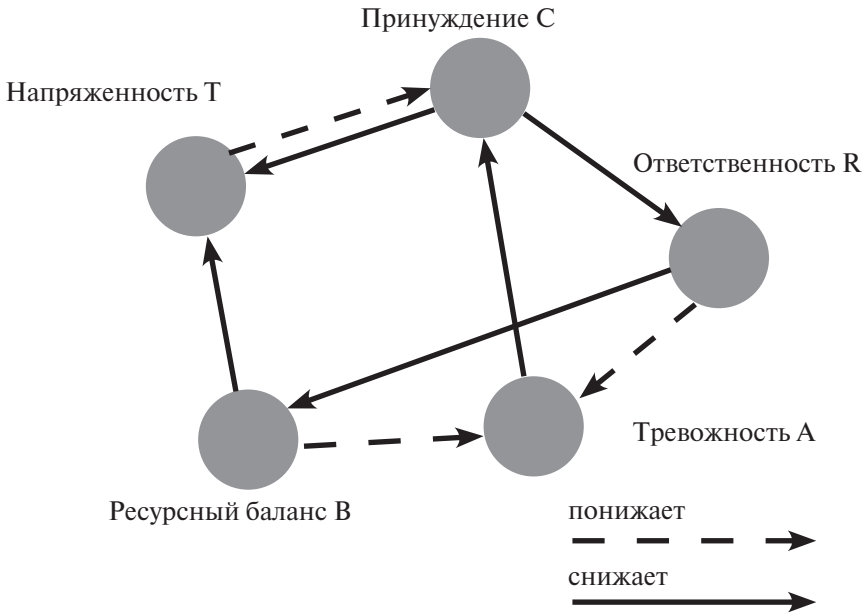
Рис. 8. Тренд-структура связей между основными переменными кольцевой динамики
