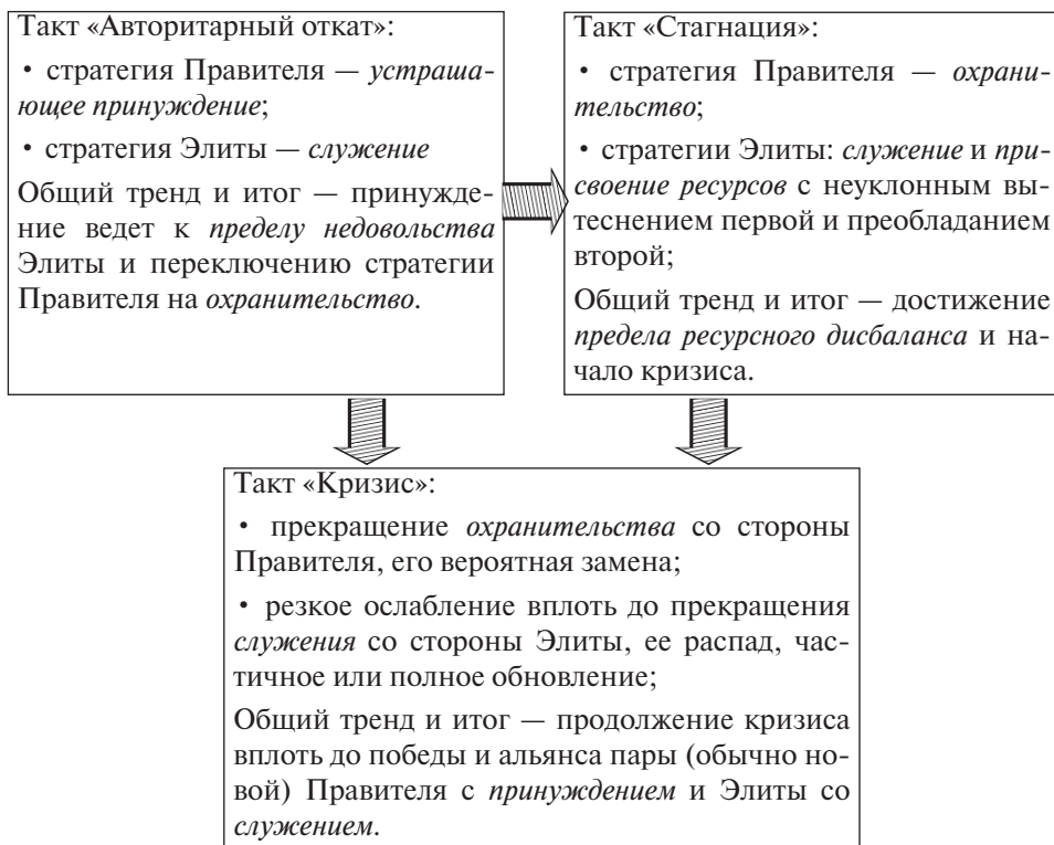
Рис. 2. Модель фазовых переходов для двух акторов с переключением их стратегий
