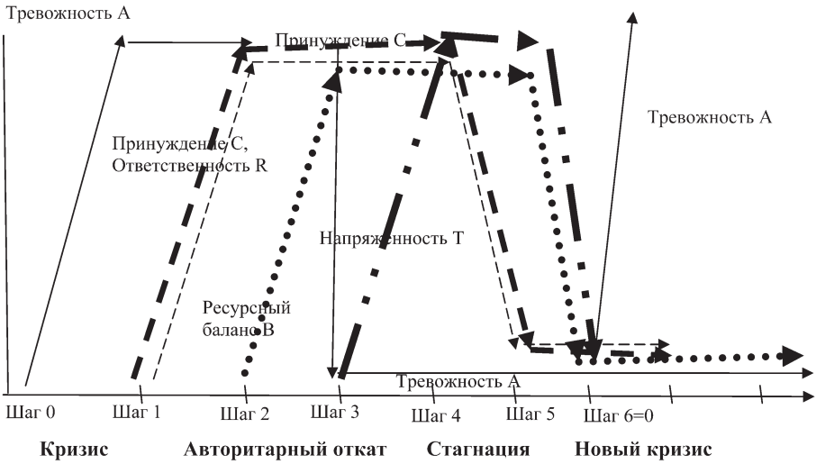
Рис. 5. График изменения значений переменных согласно постулированным правилам
