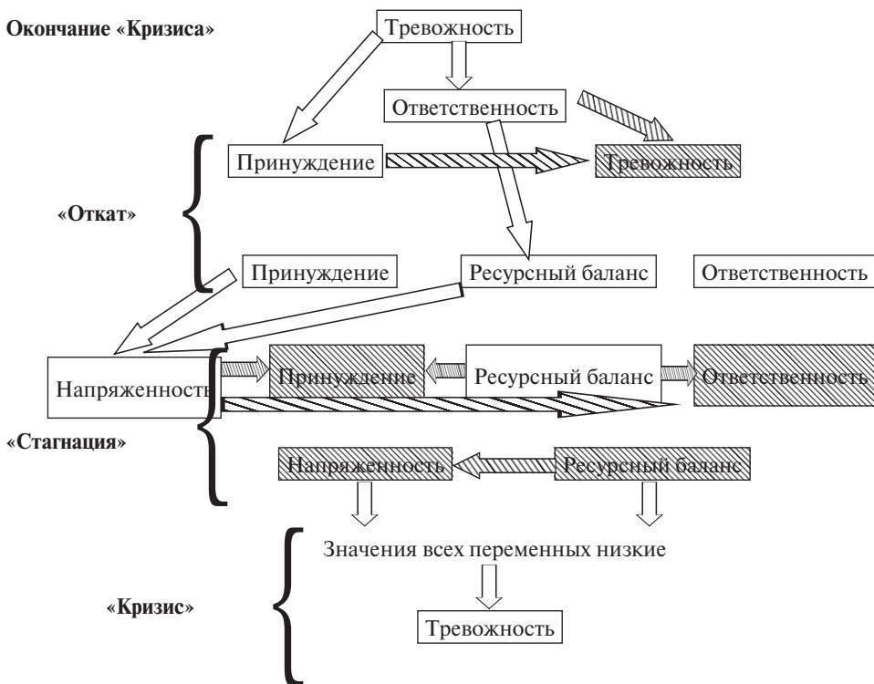
Рис. 4. Схема переключения значений бинарных переменных.
