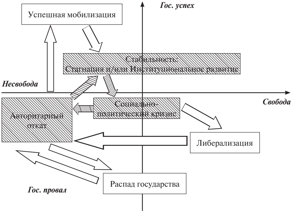
Рис. 1. Основные такты и межтакты переходы в циклической динамике истории России.
