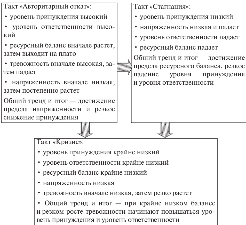
Рис. 3. Состояние переменных и тенденции их изменения в каждом такте кольцевой динамики
