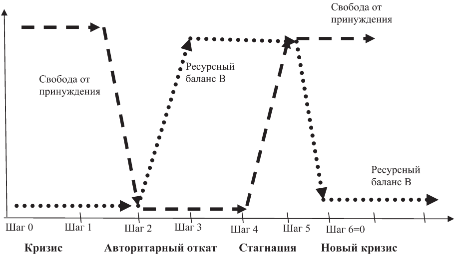
Рис. 6. Полученная средствами дискретного моделирования динамика ресурсного баланса и свободы от принуждения. Очевидна противофаза
